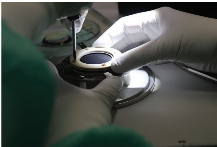
Montáž experimentálního detektoru ionizujícího záření.
